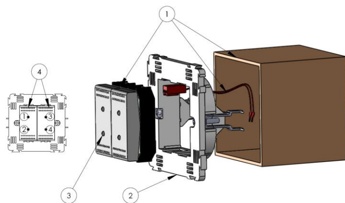
Figuur 2 : Aansluiting Bticino® schakelaar SWC04.
