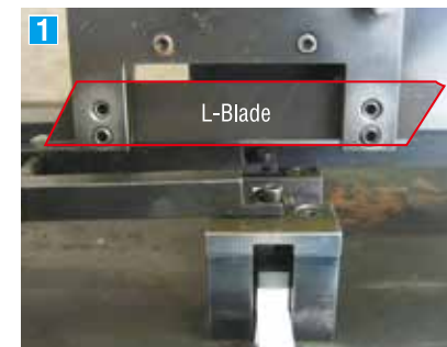
Step 1 : Setting up a blade
